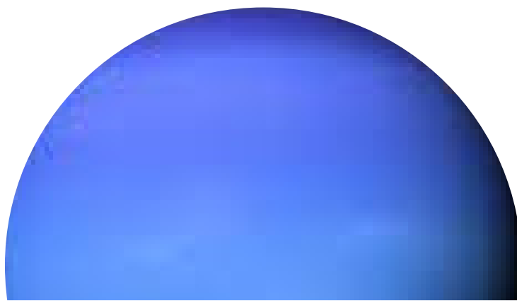
Neptú
