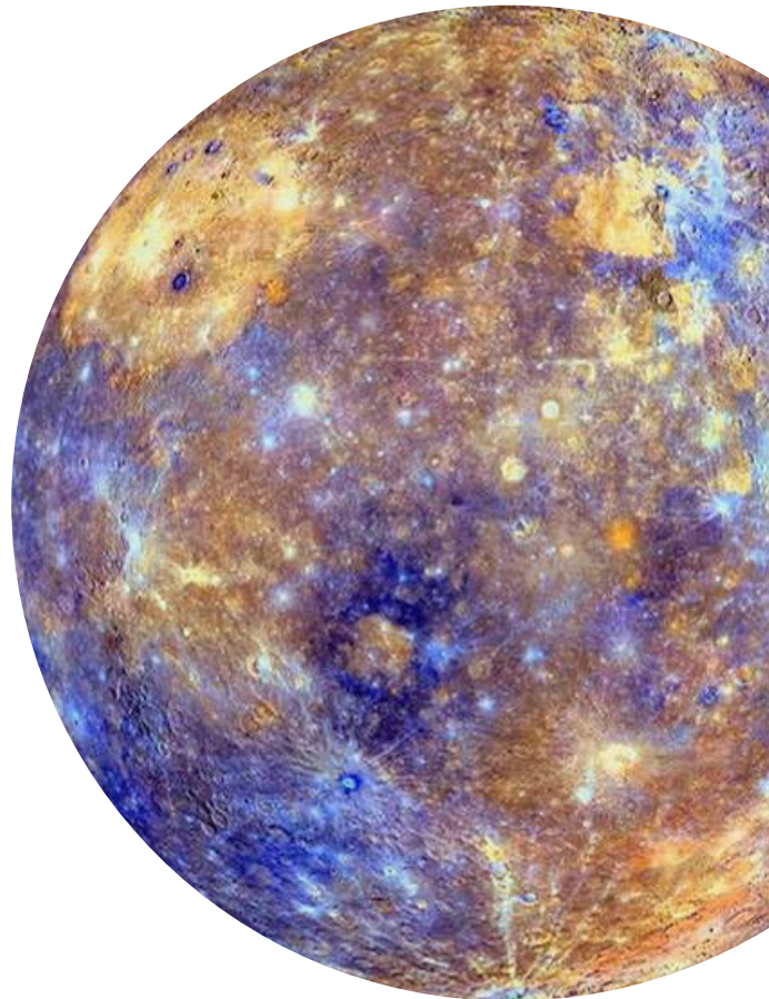
Mercur
